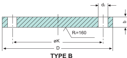
PN 40
